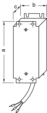
Выходной дроссель для типоразмера A 6SE6400-3TC00-4AD2 6SE6400-3TC00-4AD3
