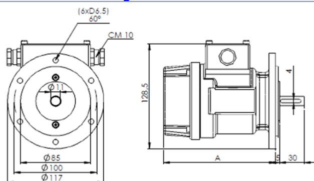
RE.0444R – B5 flange
