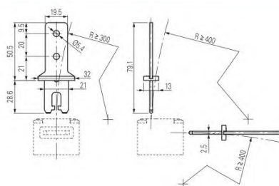
Actuator VF KEYF20
