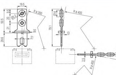
Actuator VF KEYF22
