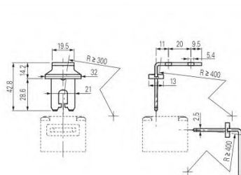
Actuator VF KEYF21
