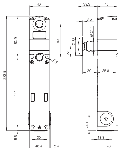
Actuator VN NG-F3•
