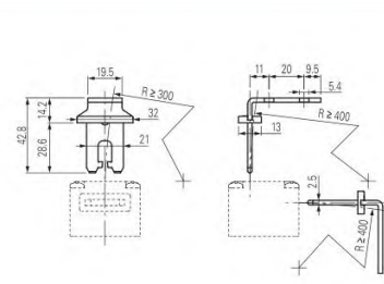
Actuator VF KEYF21
