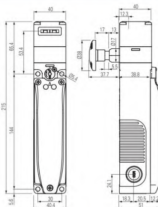
Actuator VF KEYF20
